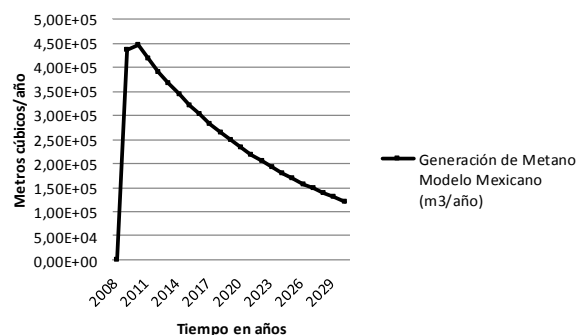
Gráfico 2. Generación de gas metano. Modelo mexicano (m 3 /año), Relleno Sanitario Doña Juana Zona II Área 3
